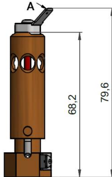
Maße R-AMFE Auslösekopf
