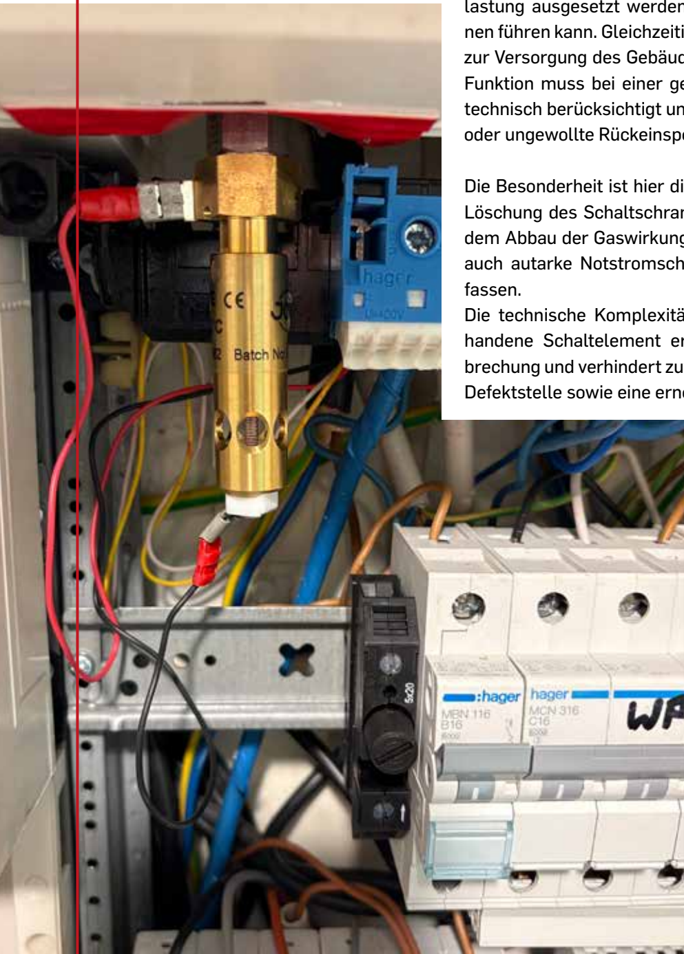
Abschaltfunktion des Schaltschrankes (u. a. für Wärmepumpe und elektrische Zusatzheizung) sowie Sperrung der Zuschaltung der Notstromversorgung aus der Speicherbatterie.
